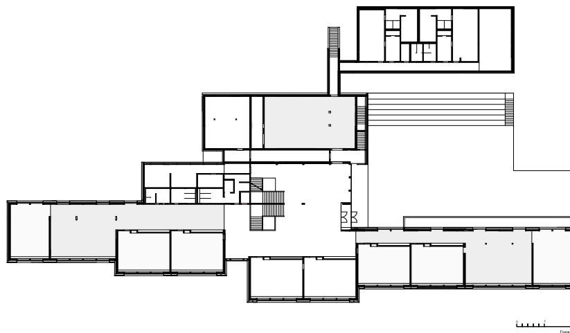
Erdgeschoß
