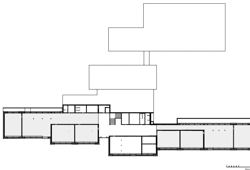
1. Untergeschoß
